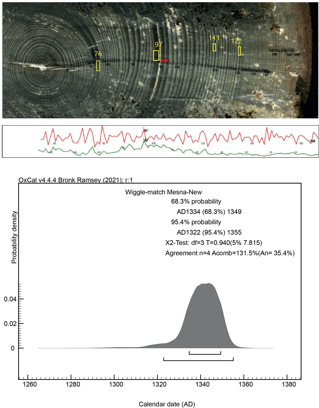
Fig. 6. Øverst: Uttak av prøver til C14-wigglematching. Skjerm bilde fra årringmålinger vha. Coorecorder (cybis.se). Nederst: Resultatet av C14-wigglematchingen av staur MSN176. – Top: Extraction of samples for C14 wiggle matching. Screenshot from annual ring measurements using Coorecorder (cybis.se). Bottom: The result of the C14 wiggle matching of pole MSN176.
