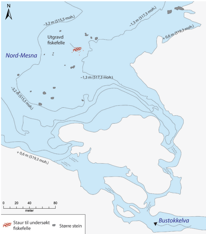
Fig. 3. Fiskefellen i Nord-Mesna var plassert om lag 100 m fra den opprinnelige strandlinjen, ved utløpet av Bustokkelva. Illustrasjon: Axel Mjørum. Det mangler dybdekart i området. Dybdelinjene er derfor basert på flyfoto på tidspunkt med ulike vannstand. – The fish trap in Nord-Mesna was located about 100 m from the original shoreline, at the outlet of the river Bustokkelva. There is a lack of depth maps for the area. The depth lines are therefore based on aerial photographs at times with different water levels.
