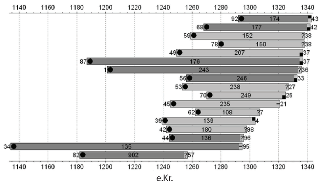
Fig. 7. Prøvene. Stolper: målte årringer med kortdato for første og siste årring. Mørk: prøver som også enkeltvis er datert mot Håckren-kronologien; lys grått: innbyrdes datert. Punkt: marg på prøven. Barkkant firkant nede = sommerved, firkant oppe = vårved, ? = usikker/mulig, strek = mangler (slitt/nedbrutt). – The samples. Bars: measured annual rings with short dates for the first and last annual rings. Dark: samples with individual dating towards the Håckren chronology, Jämtland; light grey: mutually dated. Point: pith preserved. Wane edge: square below = latewood, square above = earlywood, ? = uncertain/possible, dash = missing (worn/broken down).
